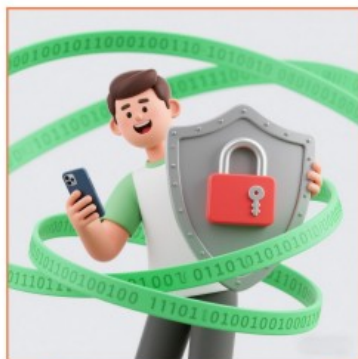
信息安全权
